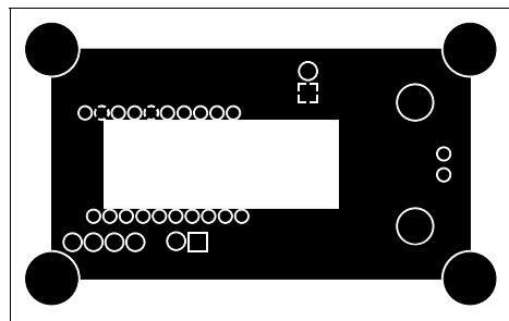
Bottom Copper Layer
