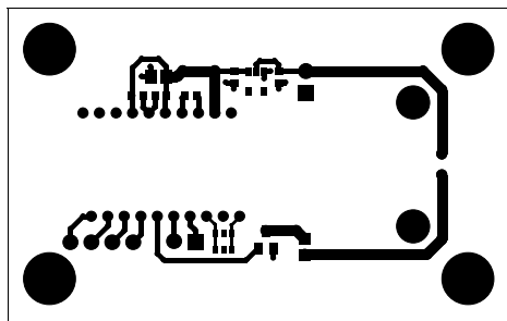
Top Copper Layer
