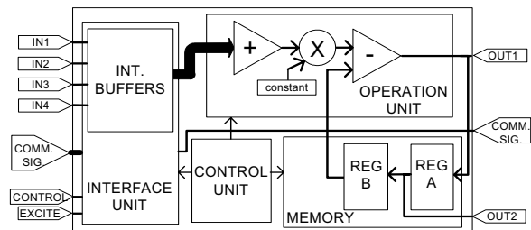
Fig. 6. Details of the PE
