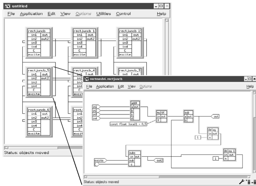
Fig. 4. GEDAE DFG of a 3X3 mesh
